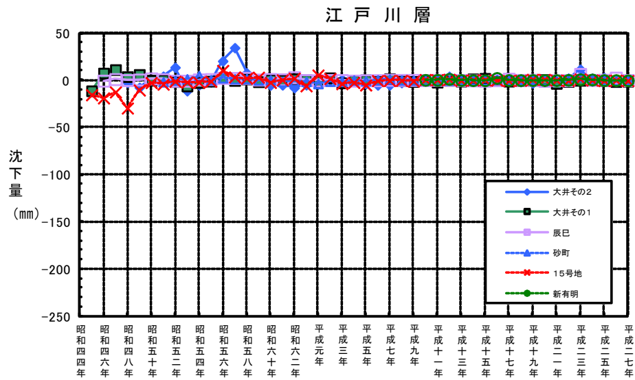
図2-2 地層毎の経年変化量(昭和45年～平成27年)
