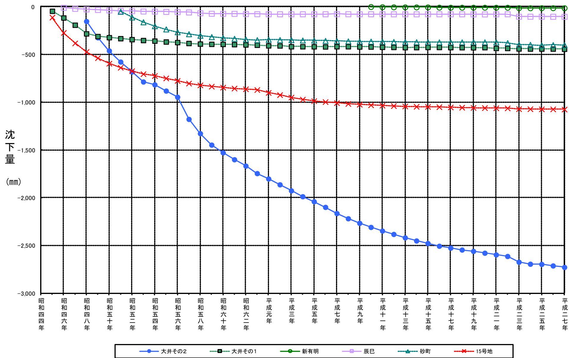
図 2 - 3 観測所毎の累計沈下グラフ (昭和 4 5 年～平成 2 7 年)
