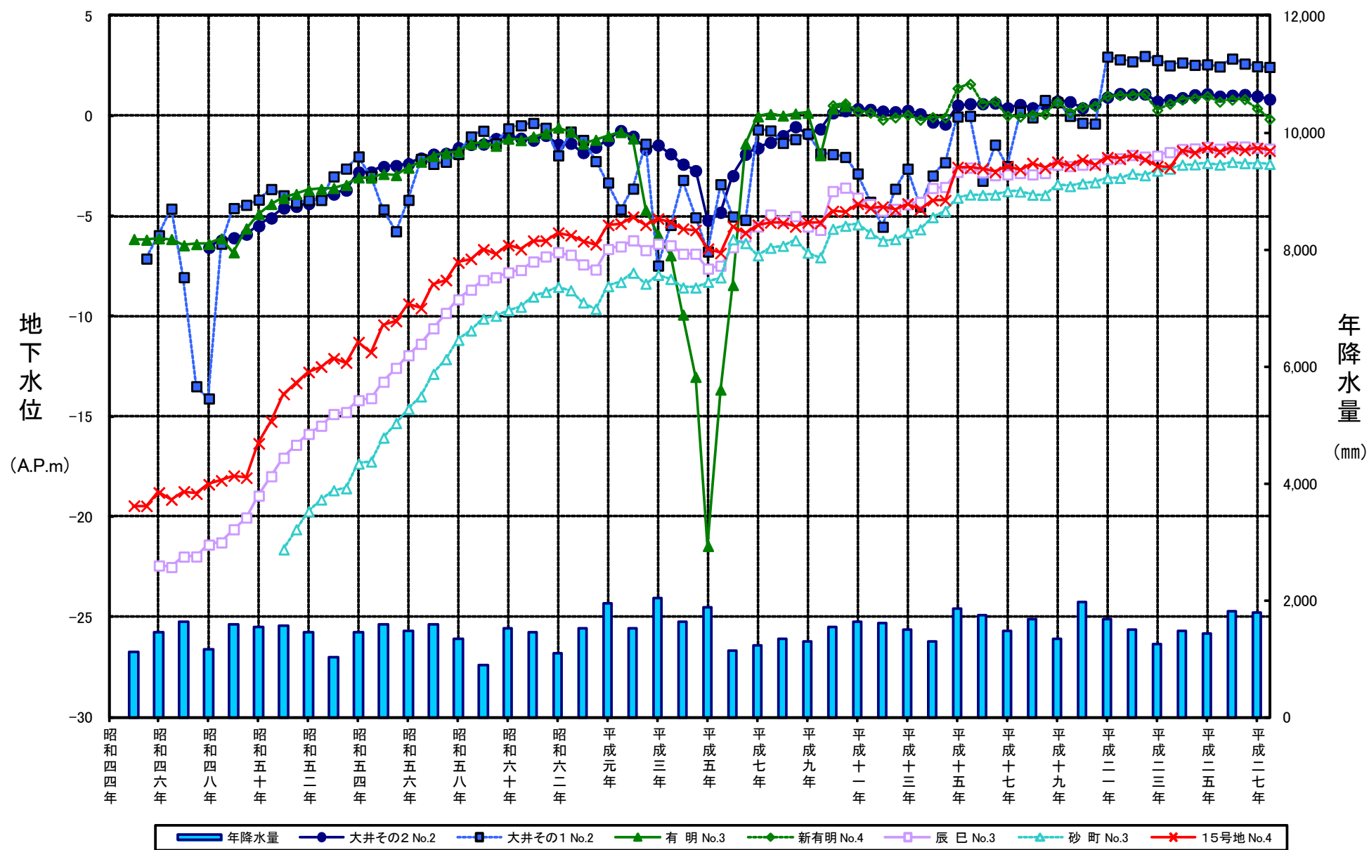
図2-4 観測所毎の地下水位変動グラフ (昭和45年～平成27年)
