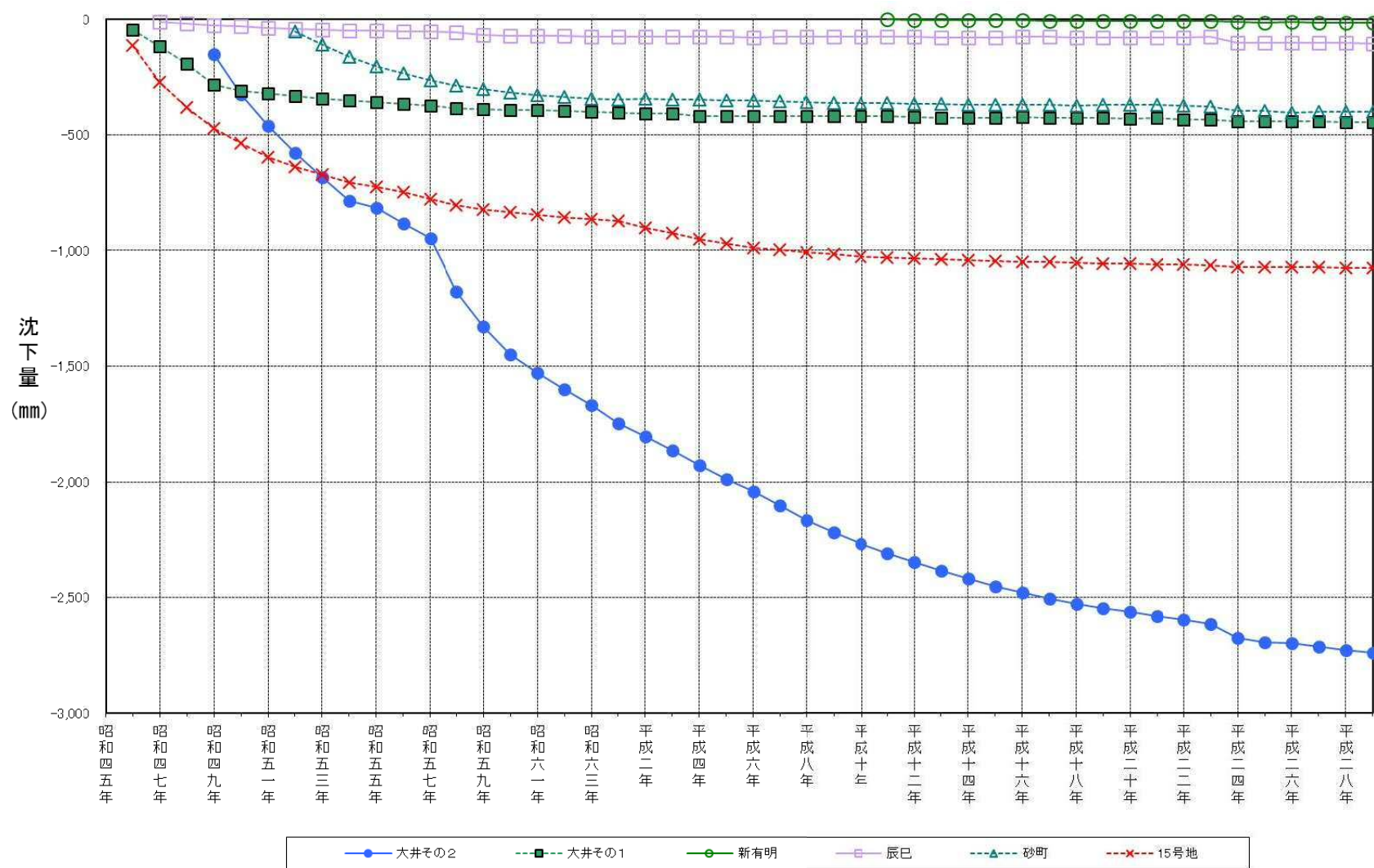
図 2 - 3 観測所毎の累計沈下グラフ (昭和 45 年～平成 28 年)
