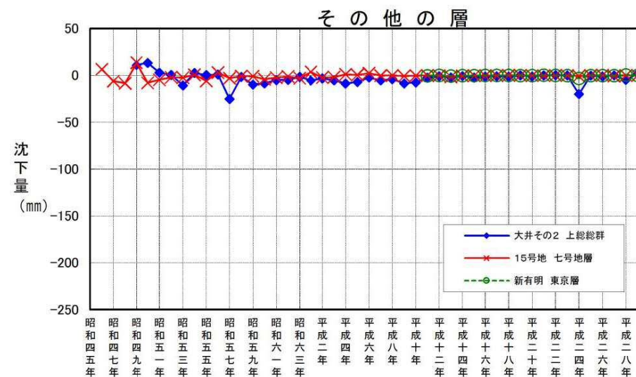
図 2 - 2 地層毎の経年変化量 (昭和 45 年～平成 28 年)
