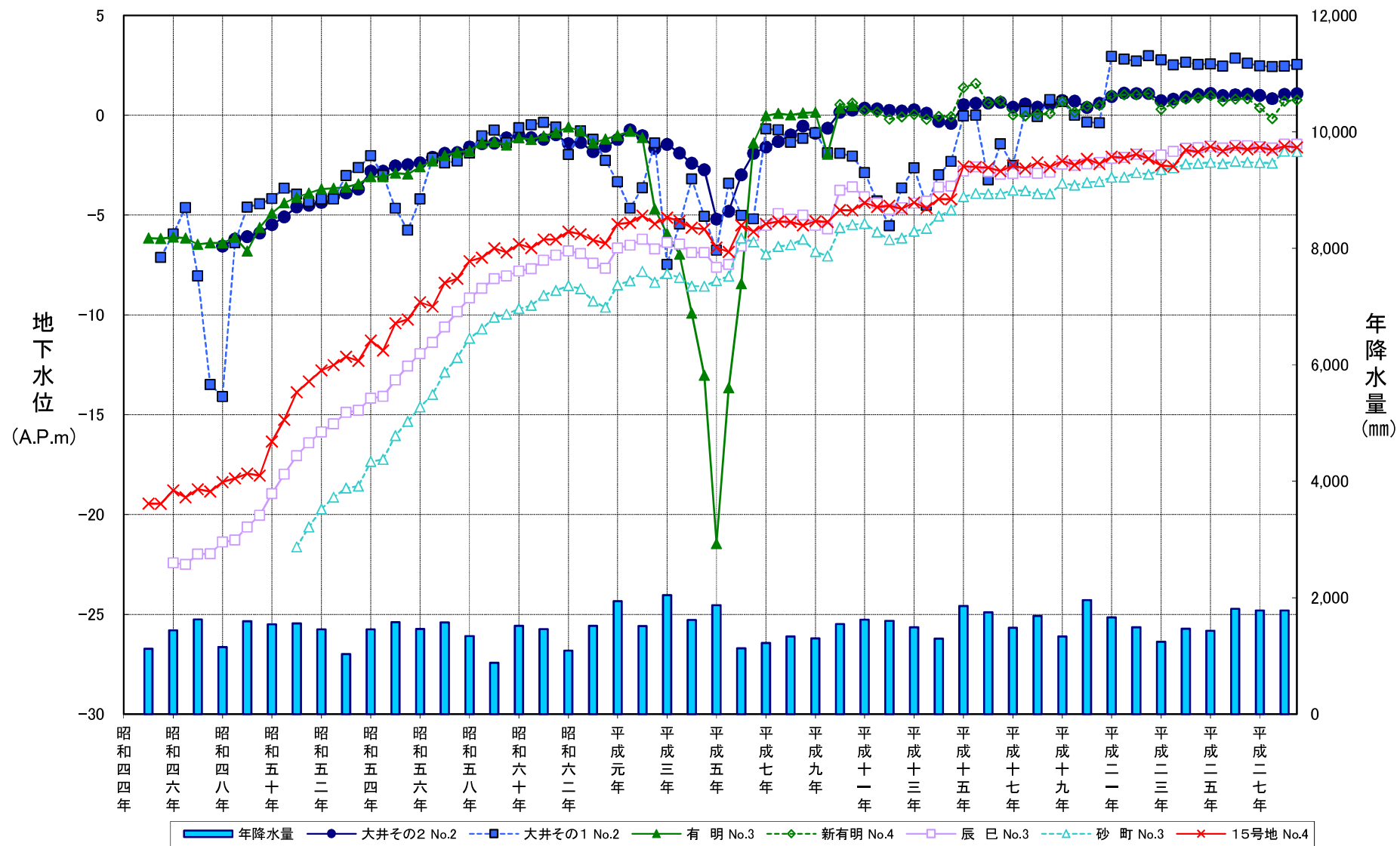
図2-4 観測所毎の地下水位変化グラフ(昭和45年～平成28年)
