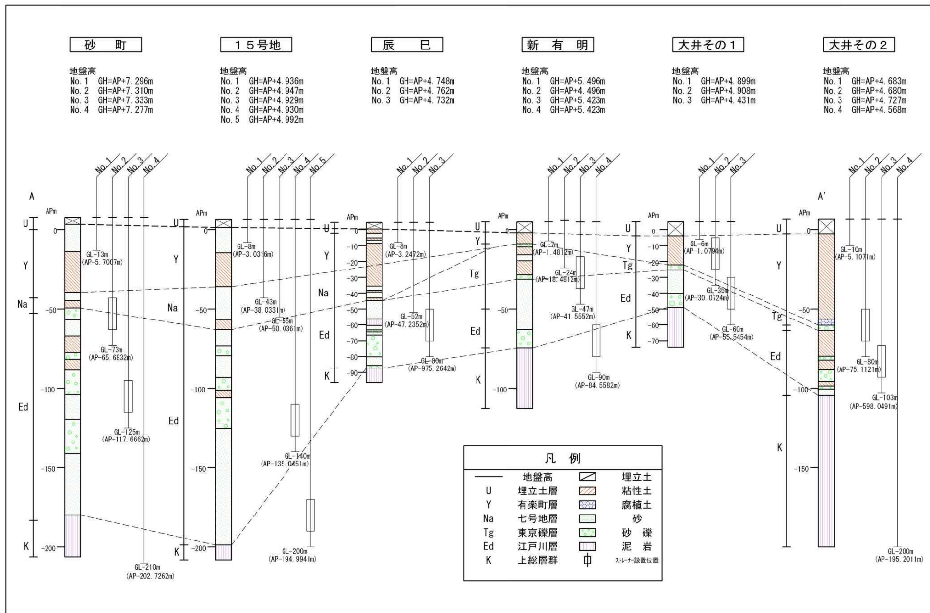
図 1-2 各観測所における観測井の深さ
