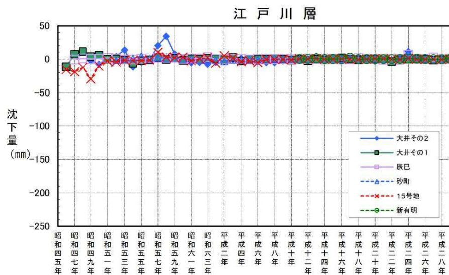
図 2 - 2 地層毎の経年変化量 (昭和 45 年～平成 28 年)
