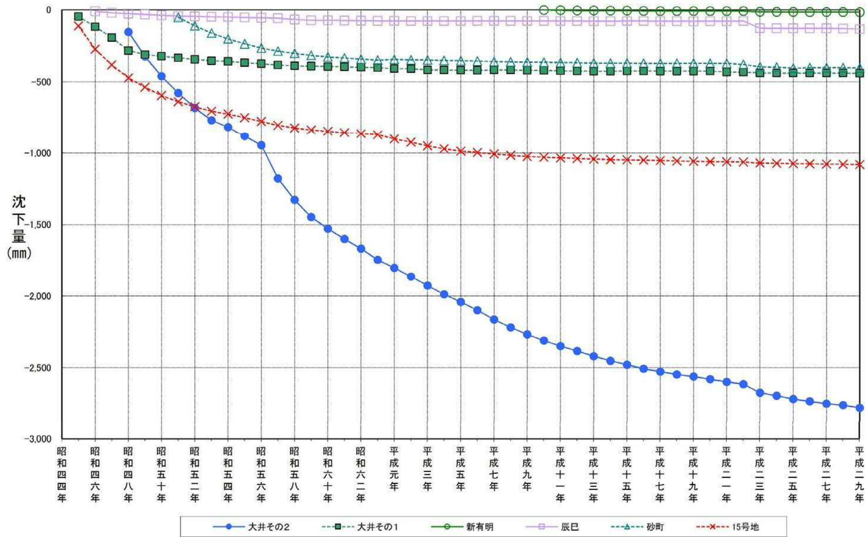
図 2 - 3 観測所毎の累計沈下グラフ (昭和 45 年～平成 29 年)
