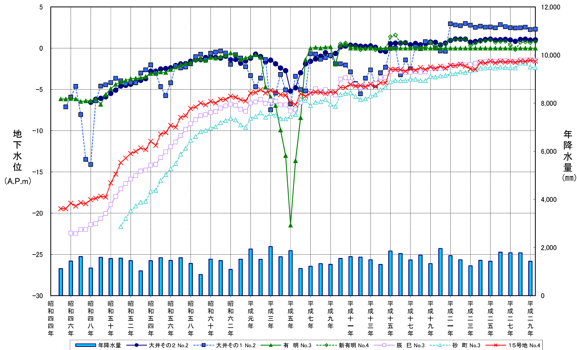
図2-4 観測所毎の地下水水位変化グラフ(昭和45年～平成29年)
