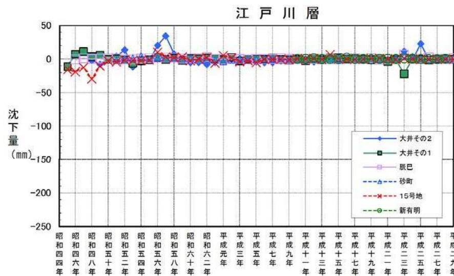
図 2 - 2 地層毎の経年変化量 (昭和 45 年～平成 29 年)
