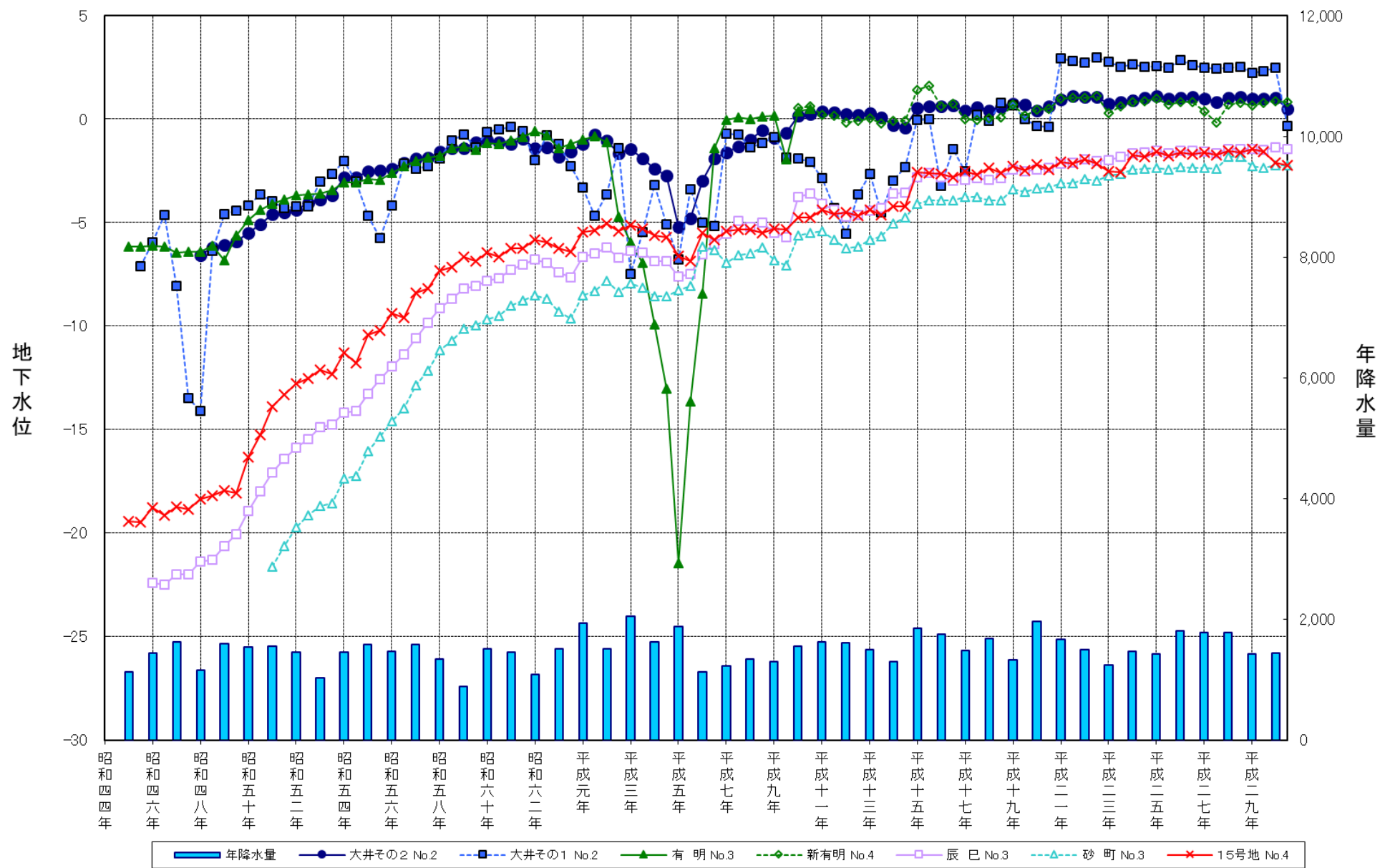
図 2 - 4 観測所毎の地下水位変動グラフ (昭和 45 年～平成 30 年)
