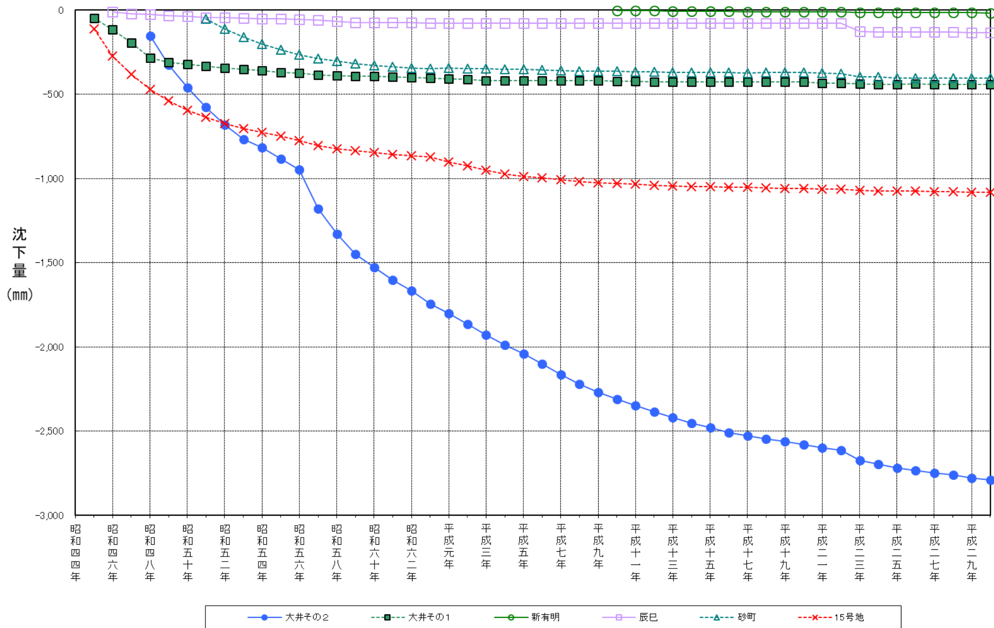
図2-3 観測所毎の累計沈下グラフ（昭和45年～平成30年）
