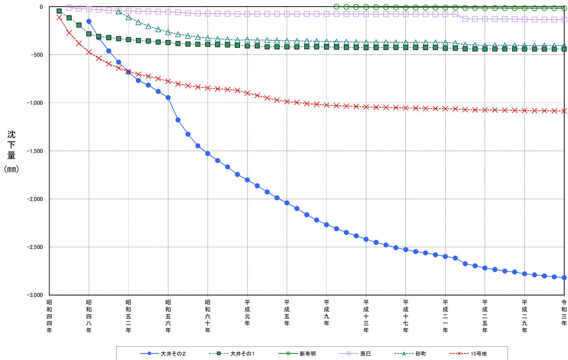
図 2 - 3 観測所毎の累計沈下グラフ (昭和 45 年～令和 3 年) * : 大井その 1・・・平成 21 年度移
