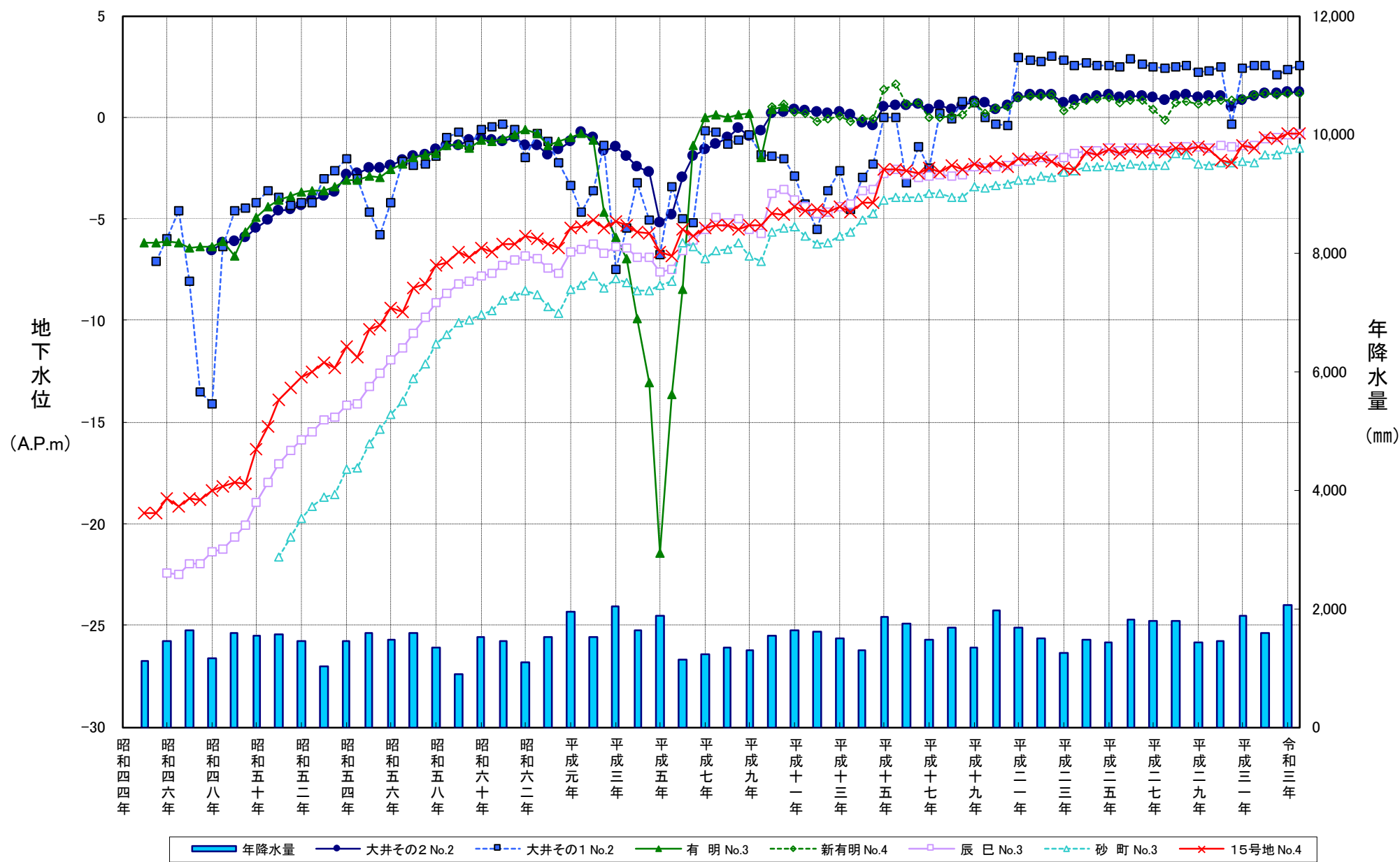
図2-4 観測所毎の地下水水位変動グラフ (昭和45年～令和3年)
