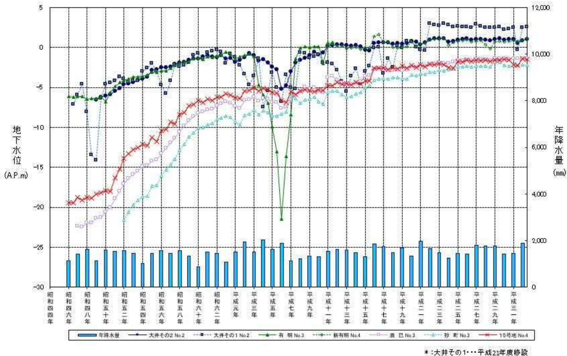
図 2 - 4 観測所毎の地下水水位変動グラフ (昭和 45 年～平成 31 年)
