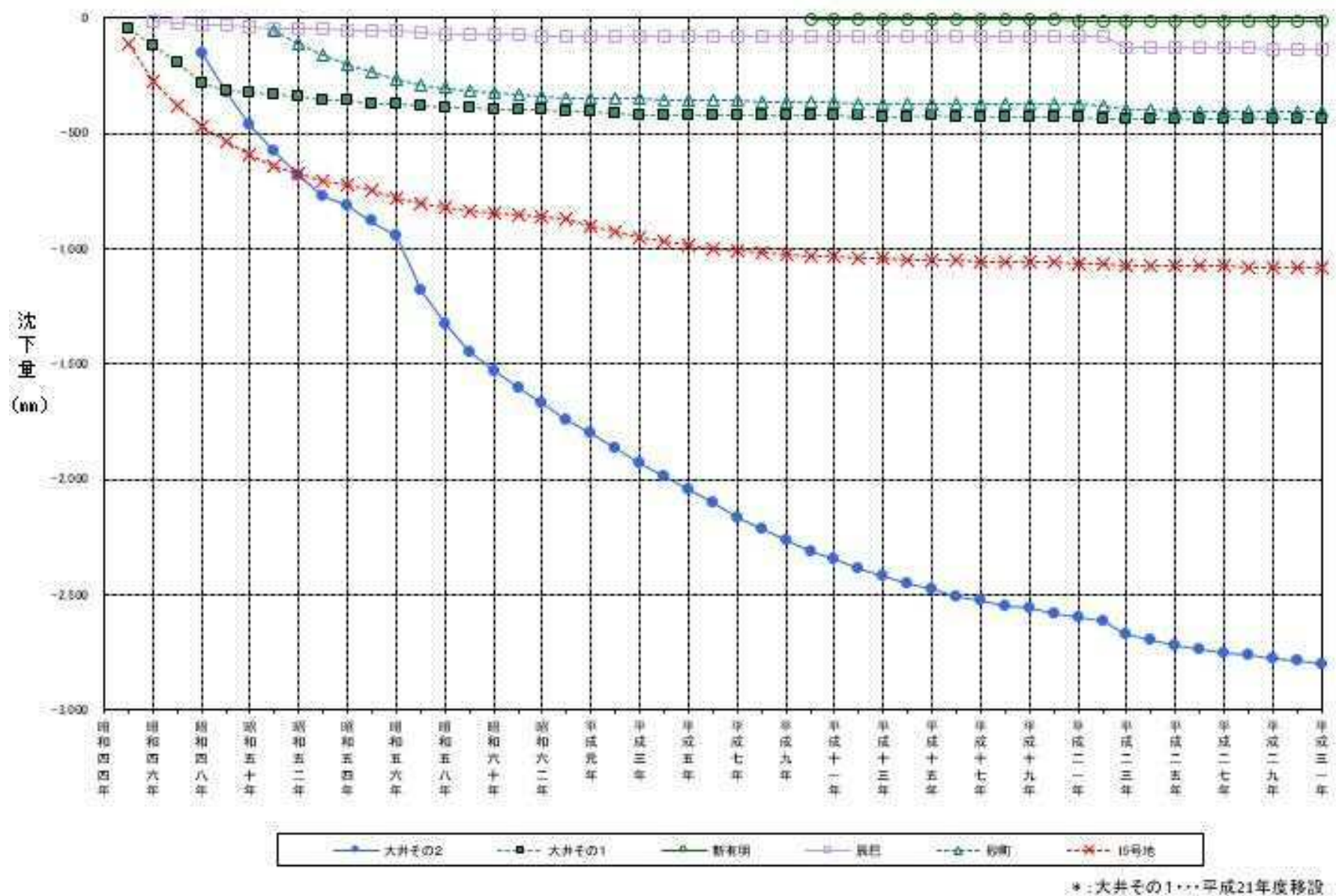
図2-3 観測所毎の累計沈下グラフ（昭和45年～平成31年）
