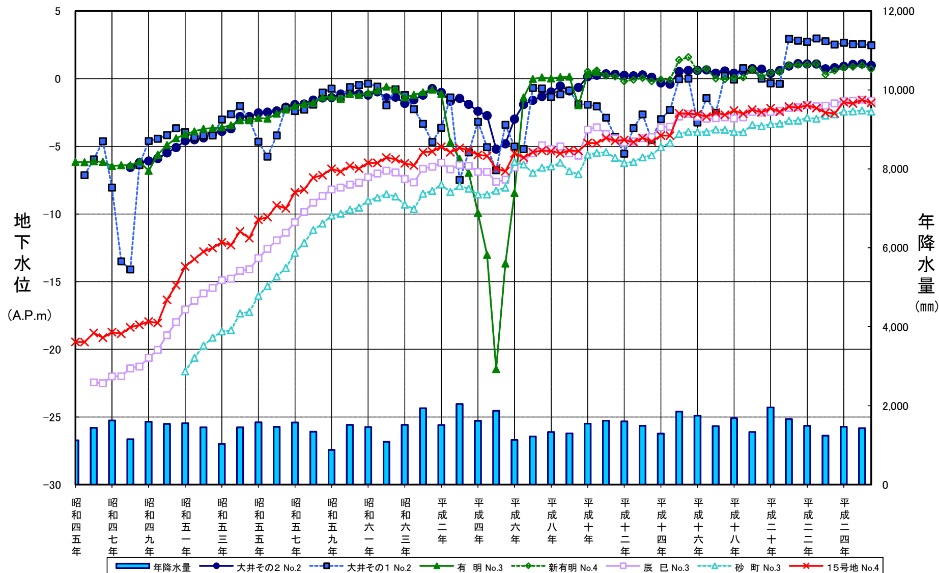
図2-4 観測所毎の地下水位変化グラフ(昭和45年～平成25年) * : 大井その1・・・平成21年度移設
