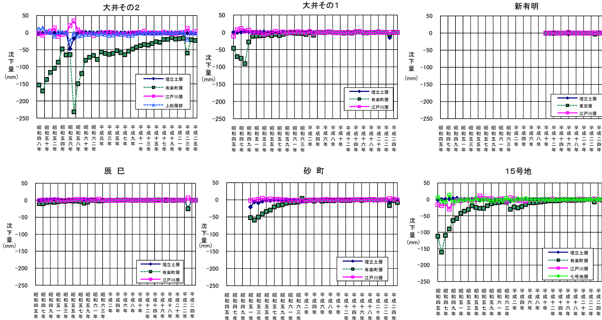
図2-1 観測所毎の経年沈下量（昭和45年～平成25年）
