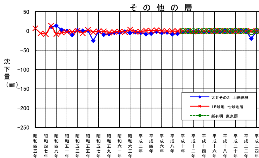
図2-2 地層毎の経年沈下量(昭和45年～平成25年)
