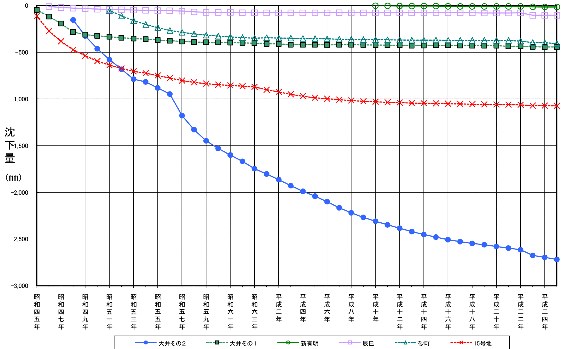
図 2 - 3 観測所毎の累計沈下グラフ (昭和 4 5 年～平成 2 5 年)
