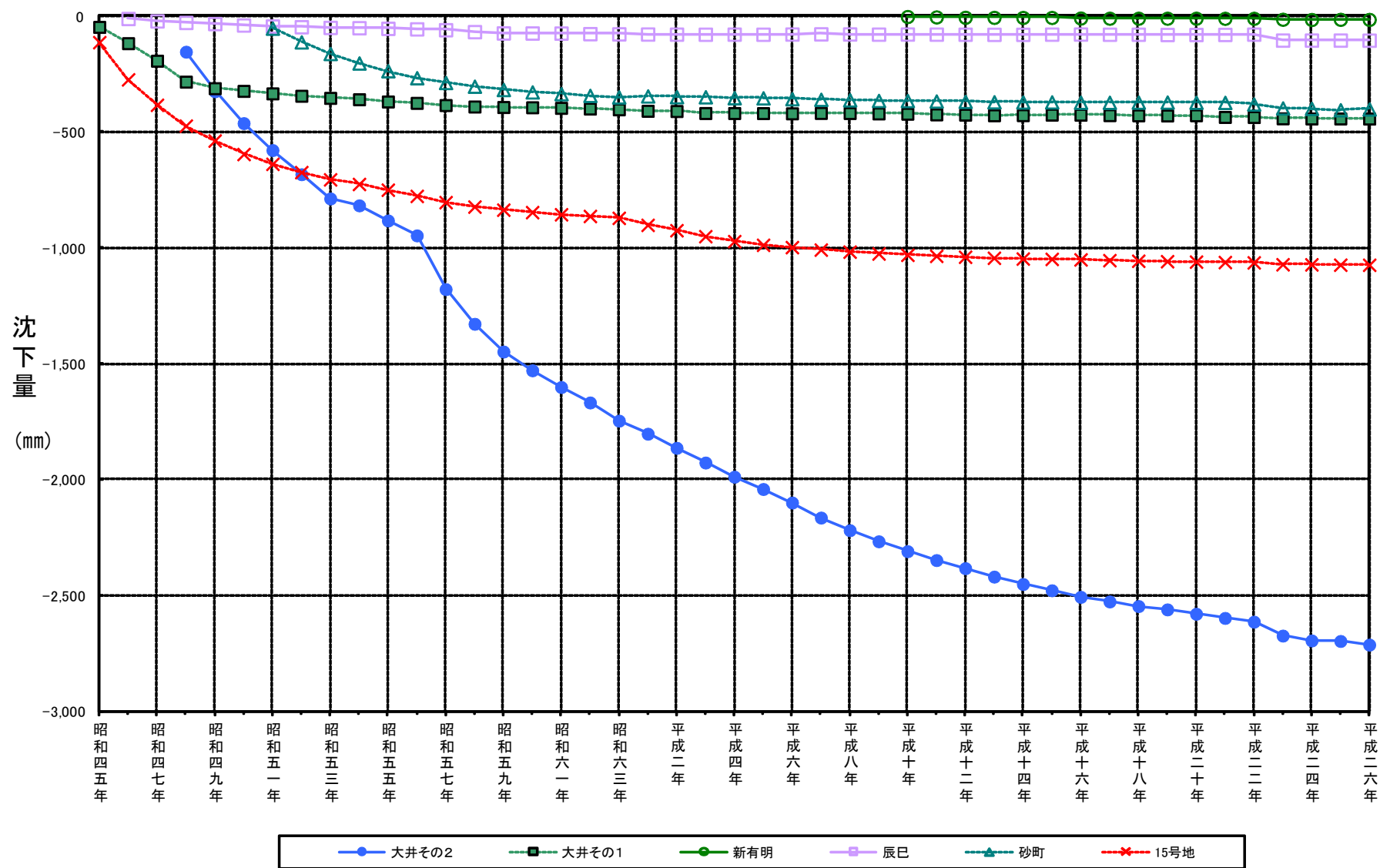
図 2 - 3 観測所毎の累計沈下グラフ (昭和 4 5 年 ~ 平成 2 6 年)
