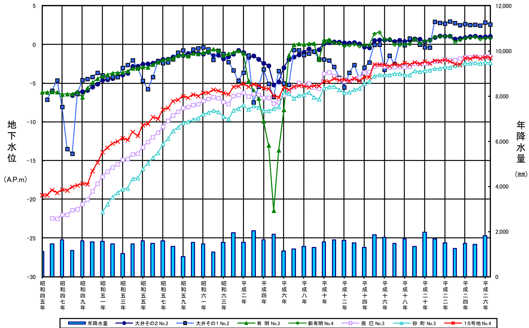
図2-4 観測所毎の地下水位変化グラフ (昭和45年～平成26年)
