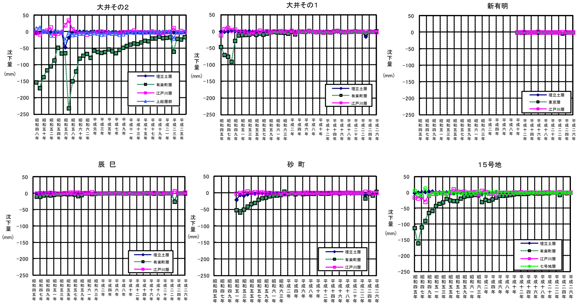
図2-1 観測所毎の経年沈下量(昭和45年～平成26年)
