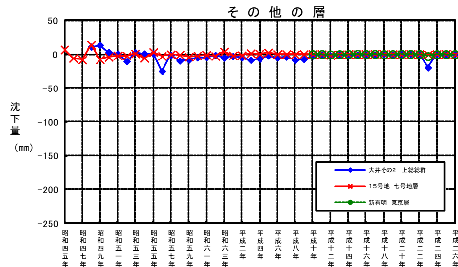
図2-2 地層毎の経年変化量（昭和45年～平成26年）
