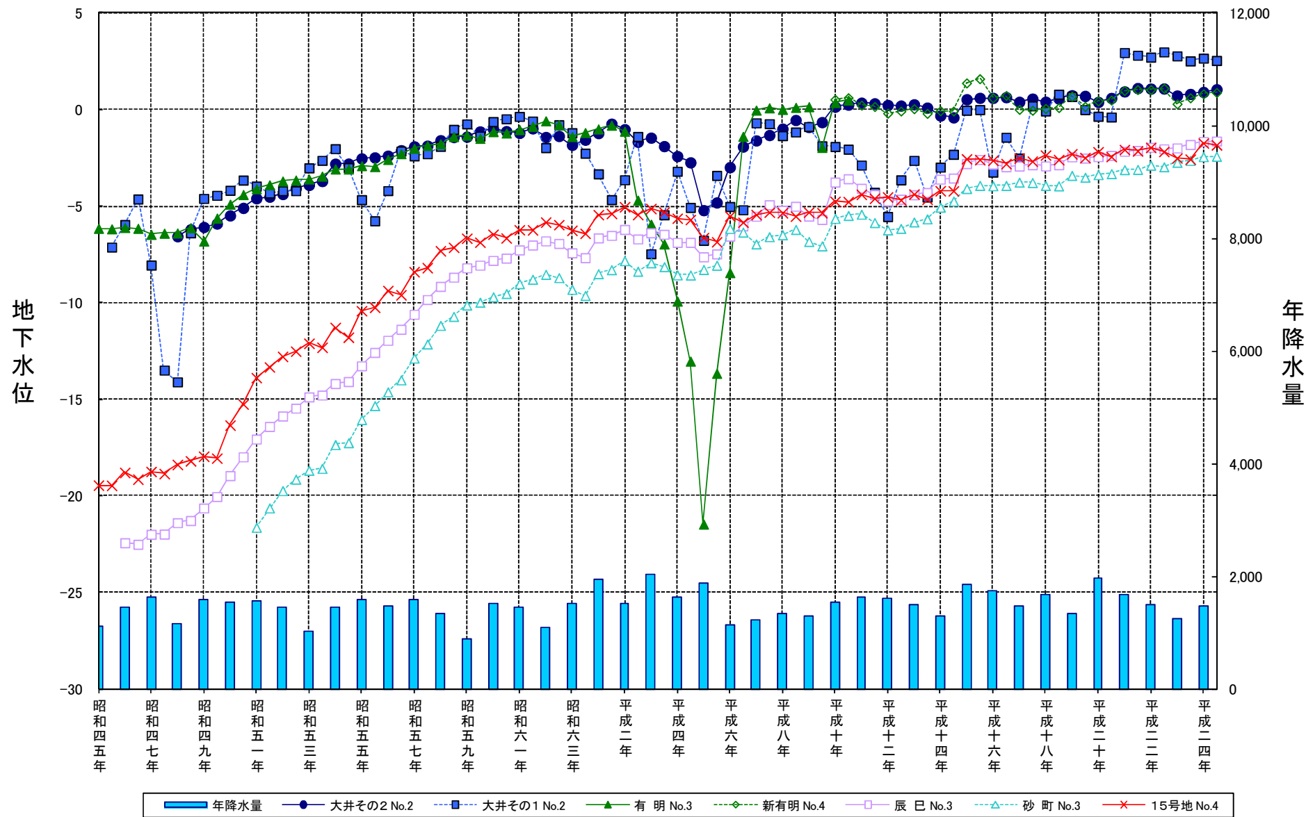
図2-4 観測所毎の地下水位変化グラフ(昭和45年～平成24年)
