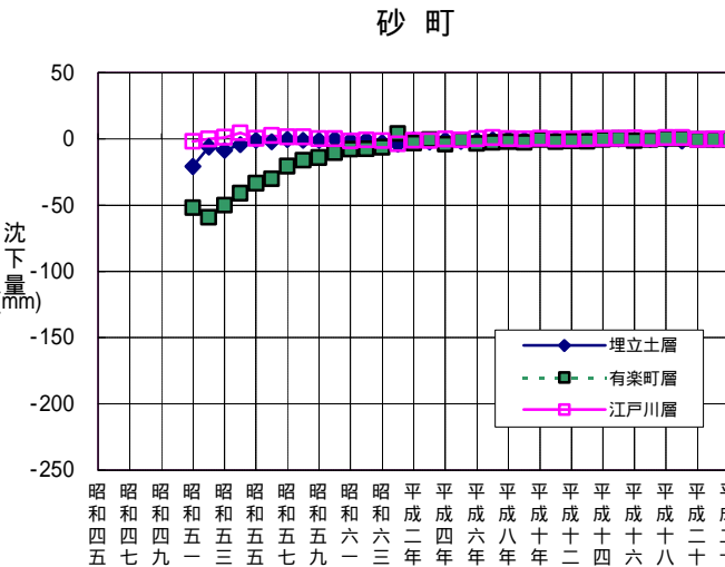
図2 - 1 観測所毎の経年沈下量 (昭和45年～平成22年)
