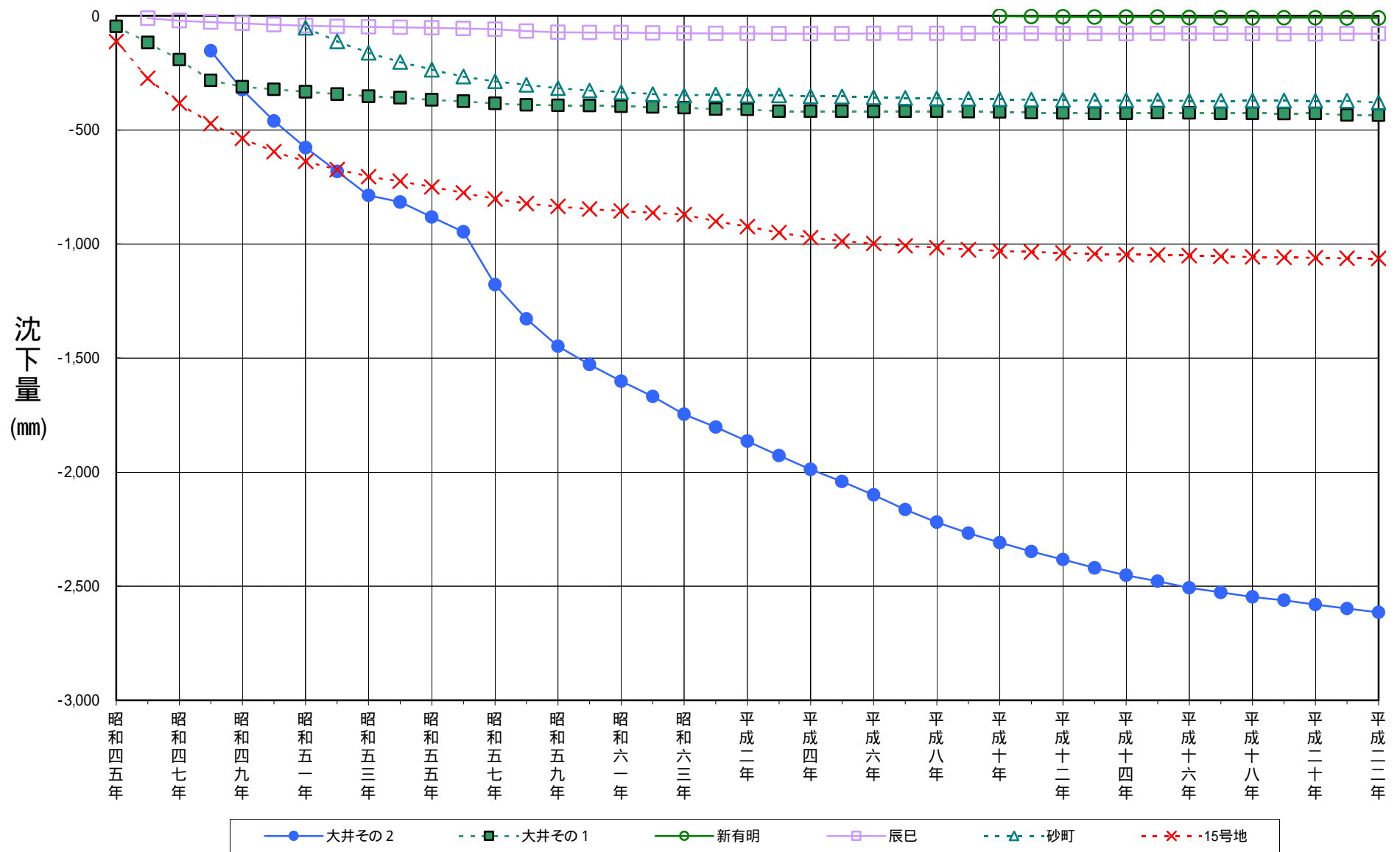
図2-3 観測所毎の累計沈下グラフ(昭和45年~平成22年)
