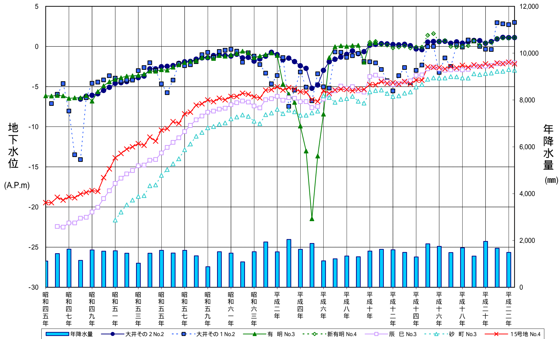
図 2- 4 観測所毎の地下水位変化グラフ (昭和 45 年 ~ 平成 22 年)
