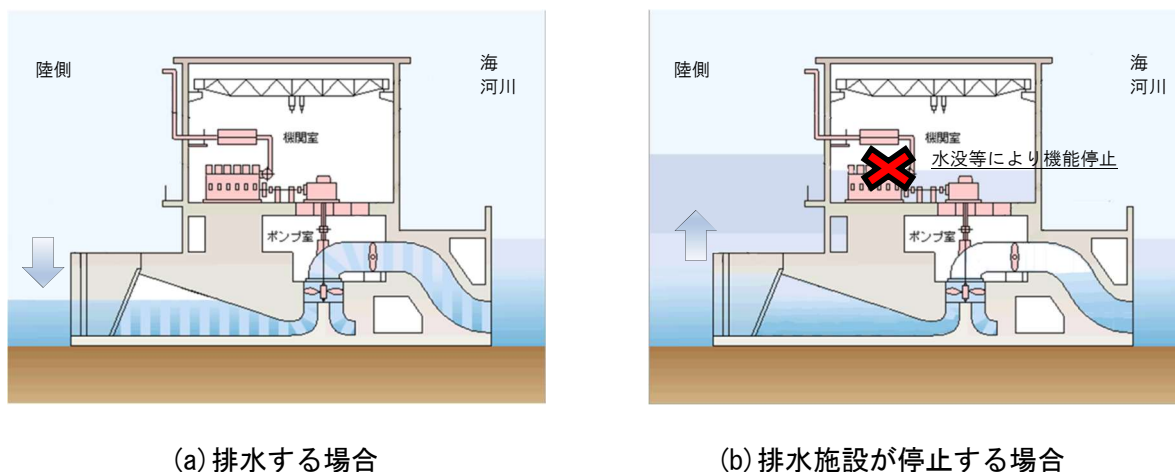
図－8 排水施設からの排水イメージ
