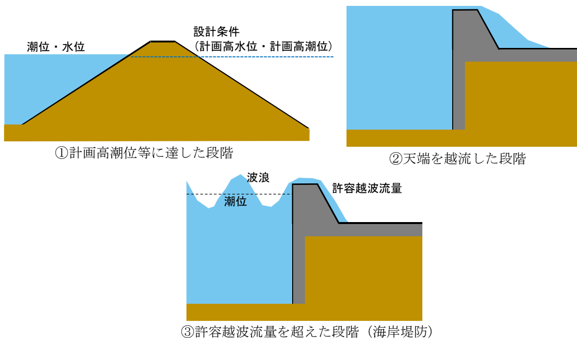
図－５ 堤防と潮位の関係（イメージ）
