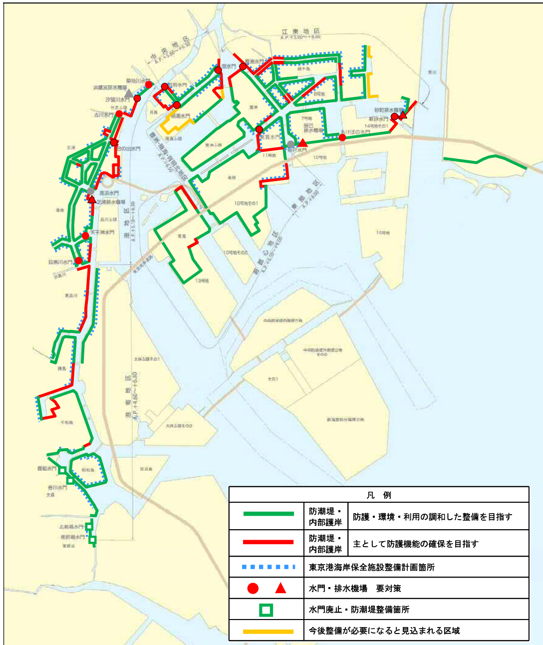
図2-1 基本計画図
