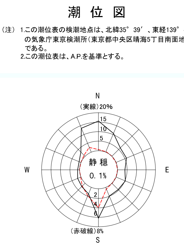
東京港風配図 平成29年(2017年)10月～令和3年(2021年)12月 観測場所:東京湾中央防波堤内側 観測回数:103,656回 (測得率:96.5%) 静穏は風速0.5m/s未満 ---は風速10m/sを超過する強風の割合を示す(8%スケール)
