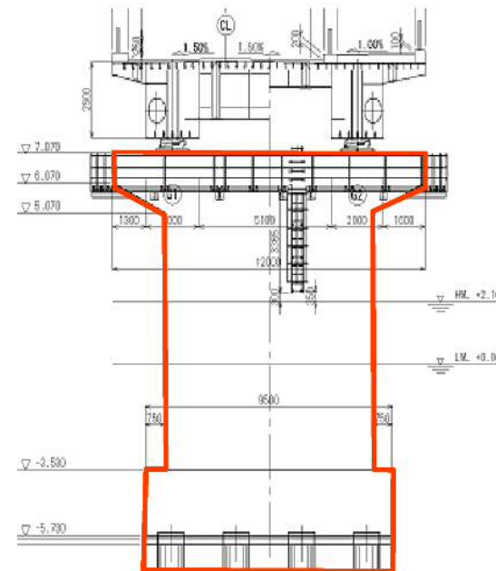
橋脚断面図
