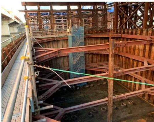
P1橋脚仮締切内状況 令和2年12月
