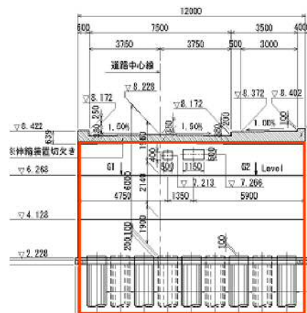
橋台断面図
