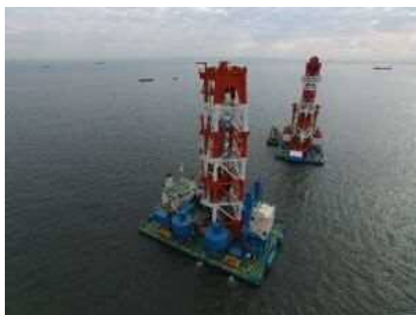
地盤改良工事（深層混合処理工） 平成30年1月
