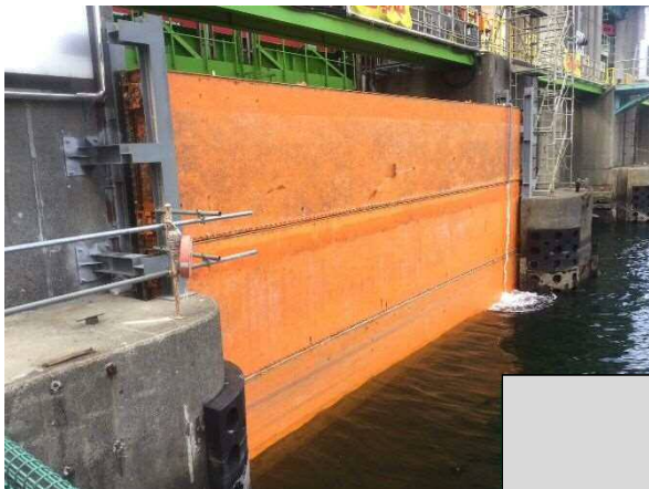
角落し設置 令和2年10月
