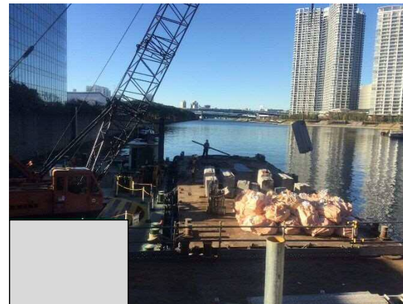
戸当り（重構造部）撤去 令和2年12月
