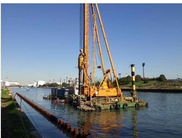
深層混合処理工 平成29年11月
