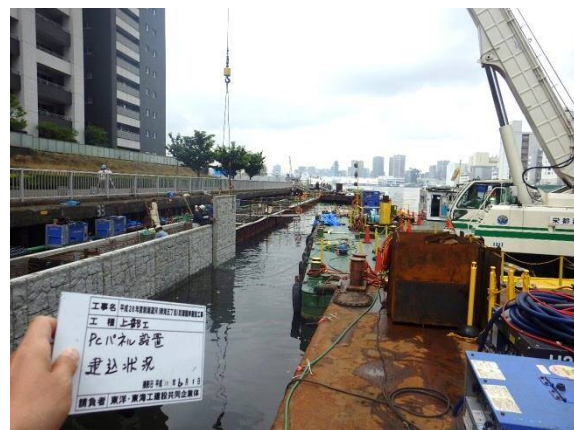
コンクリートパネル建込 平成29年6月
