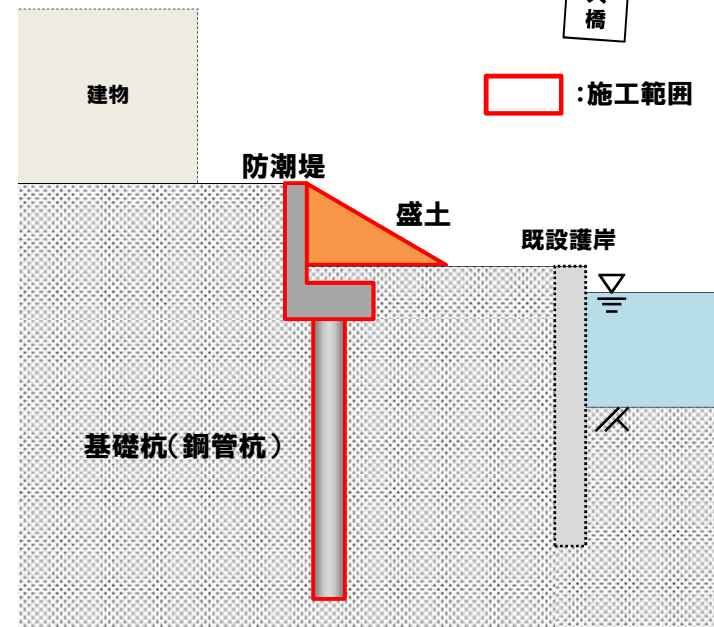
【5工区断面図】
