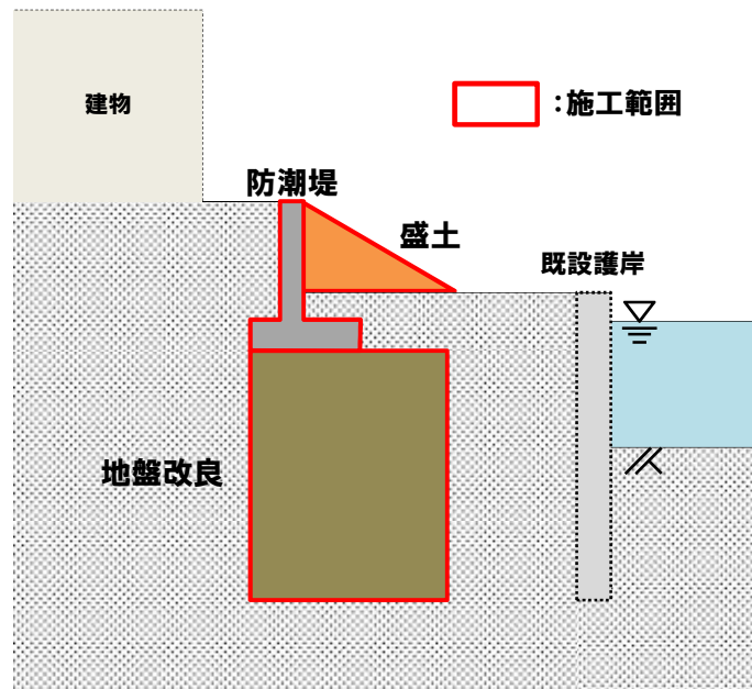
【4工区断面図】
