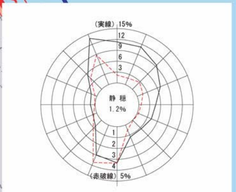
東京港風配図 昭和45年(1970年)1月~平成18年(2006年)12月 観測場所: 東京灯標 総測回数: 310,060回(測得率 96.0%) 静穏は風速0.3m/s未満 ---は風速10m/sを超過強風の割合を示す(5%スケール)
