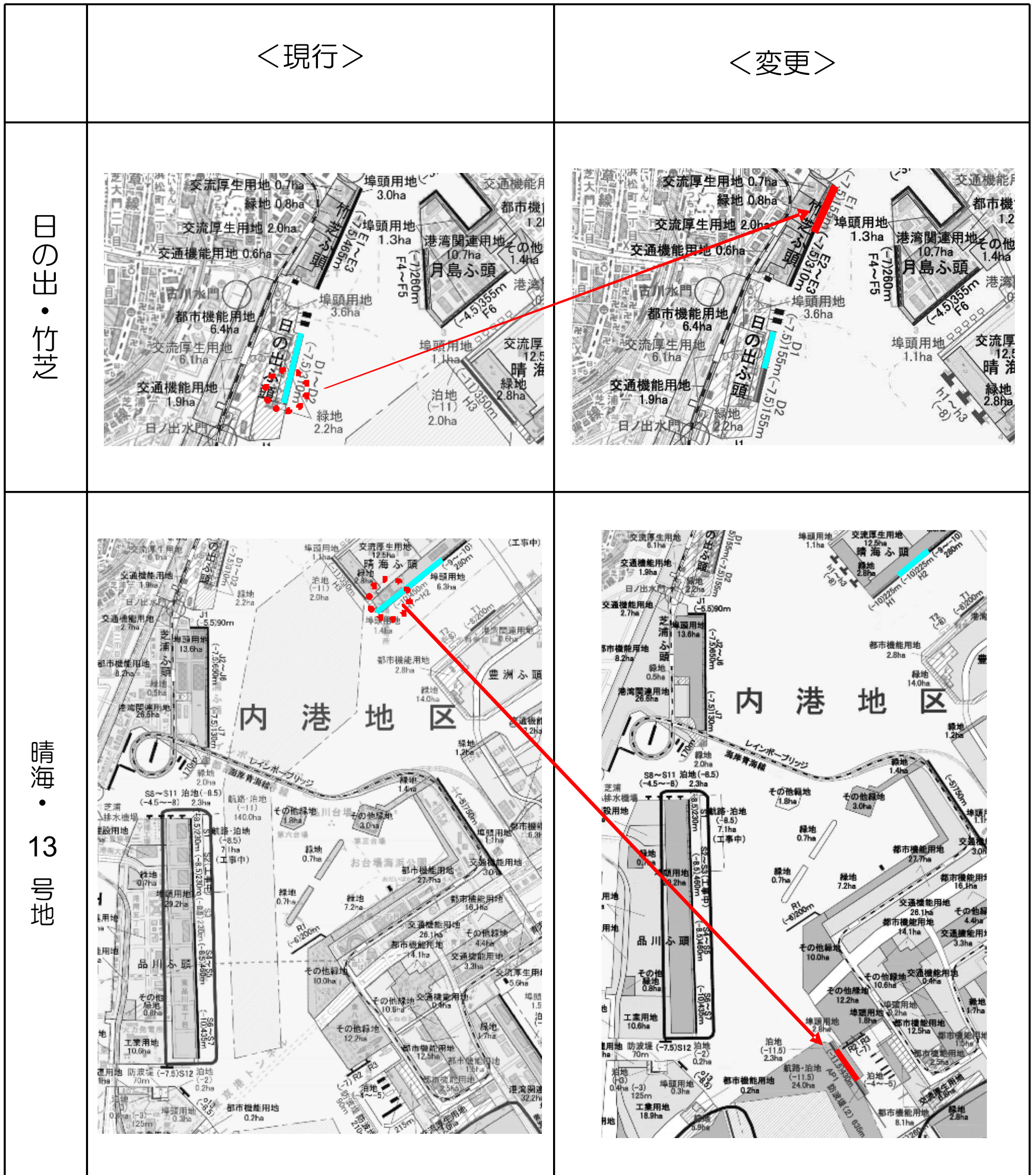
図-1 大規模地震対策施設(緊急物資輸送用耐震強化岸壁)の配置変更
