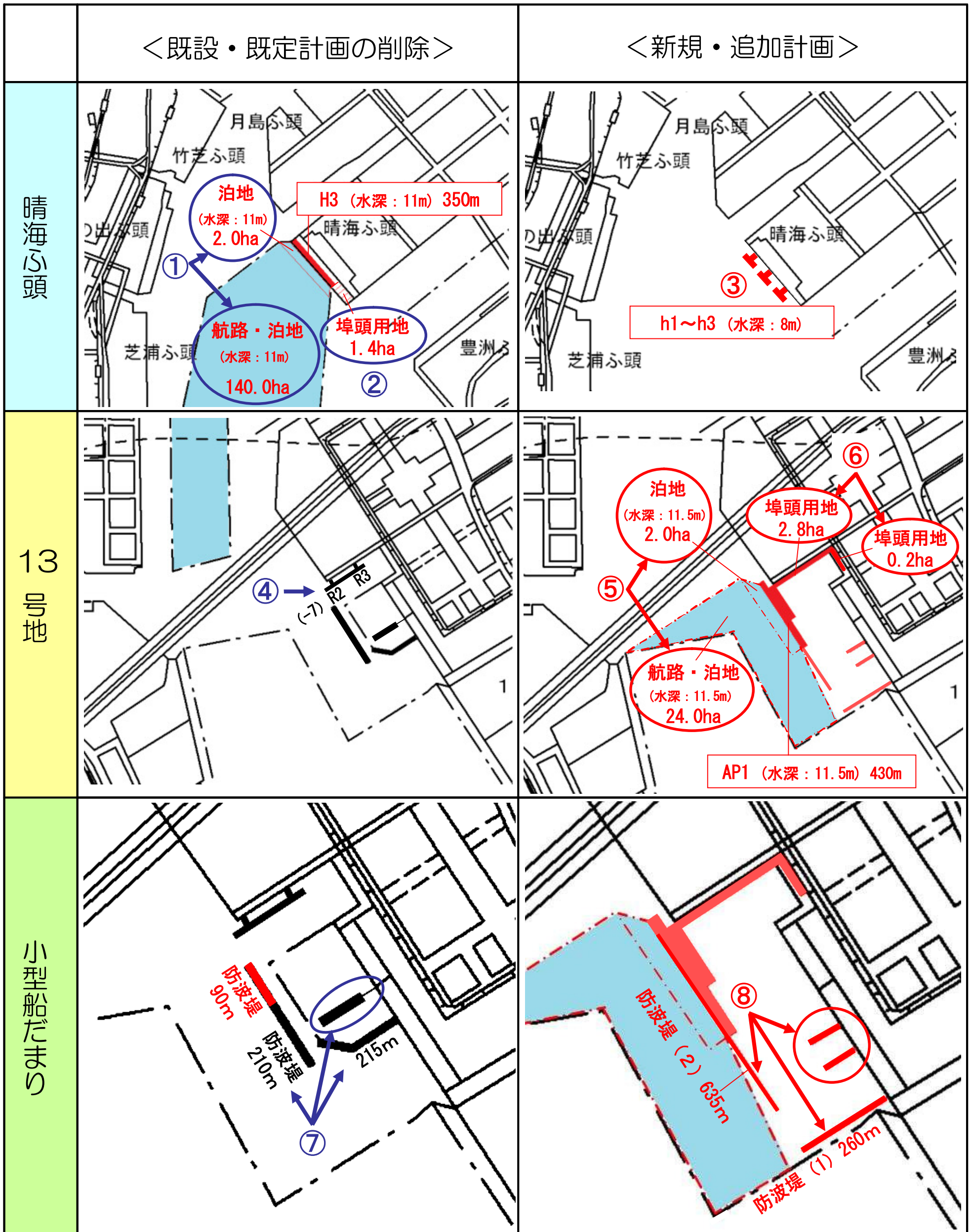
図-3 旅客船埠頭計画(大型船用)の配置変更
