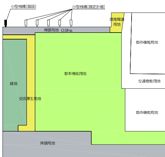
図 2-2 旅客船埠頭計画変更説明図
