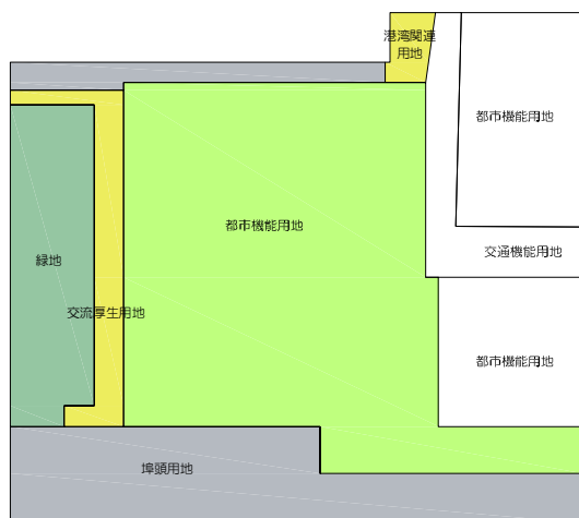
図 2-3 専用埠頭計画変更説明図
