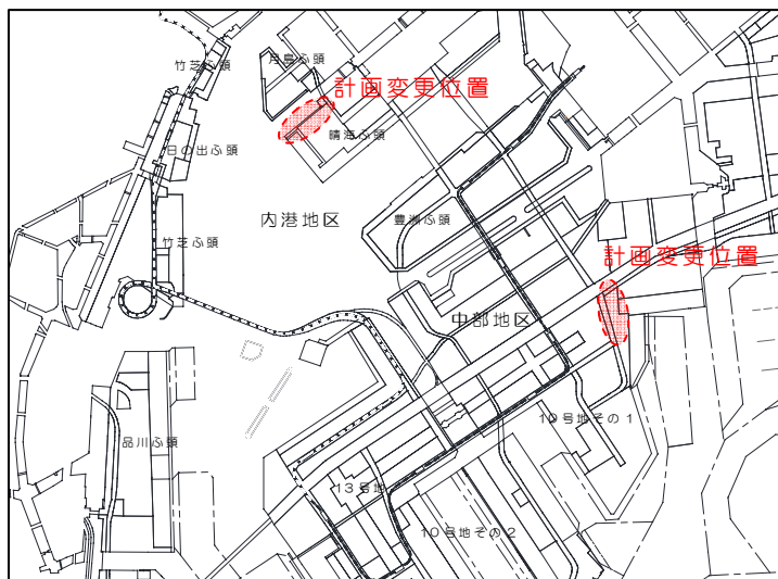
図 4-1 計画変更位置図
